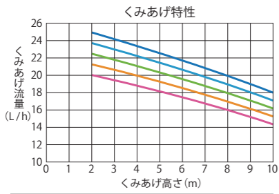
吸い上げ管横引き長さ — 0m — 10m — 20m — 30m — 40m
